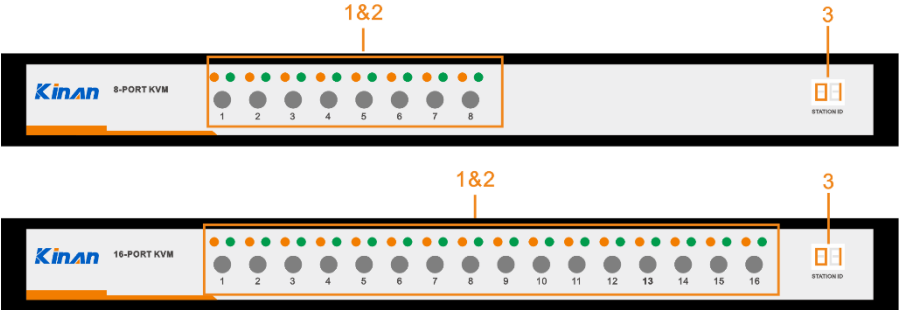
图 1.3 KVM 前视图
